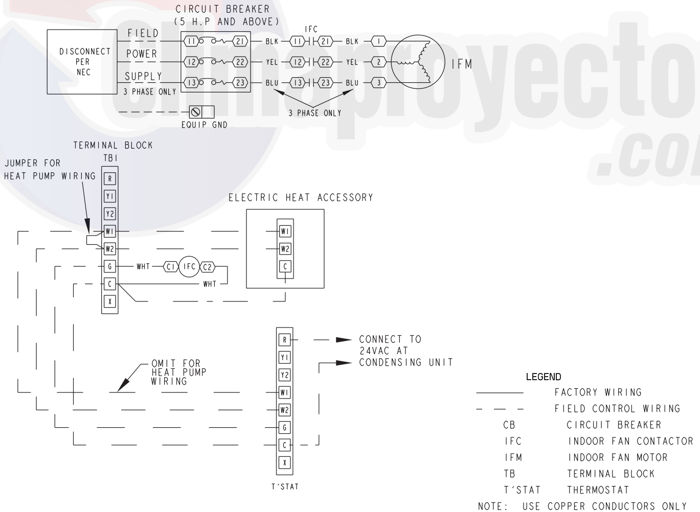
Fig. 17 - Unit Wiring
