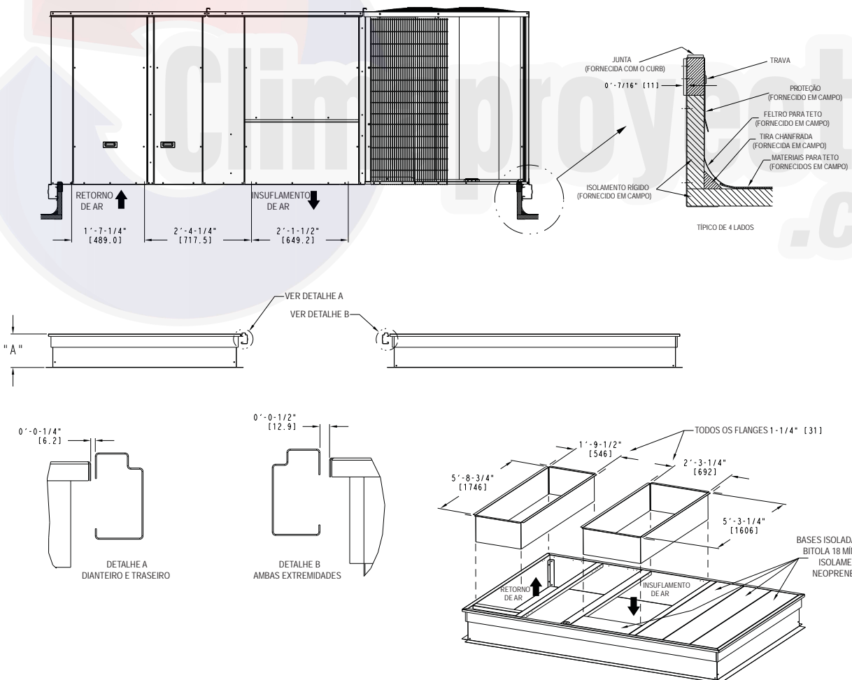
Fig. 2 (cont.) - Desenho dimensional da unidade – 50TC_20 - Detalhes do Roof Curb
