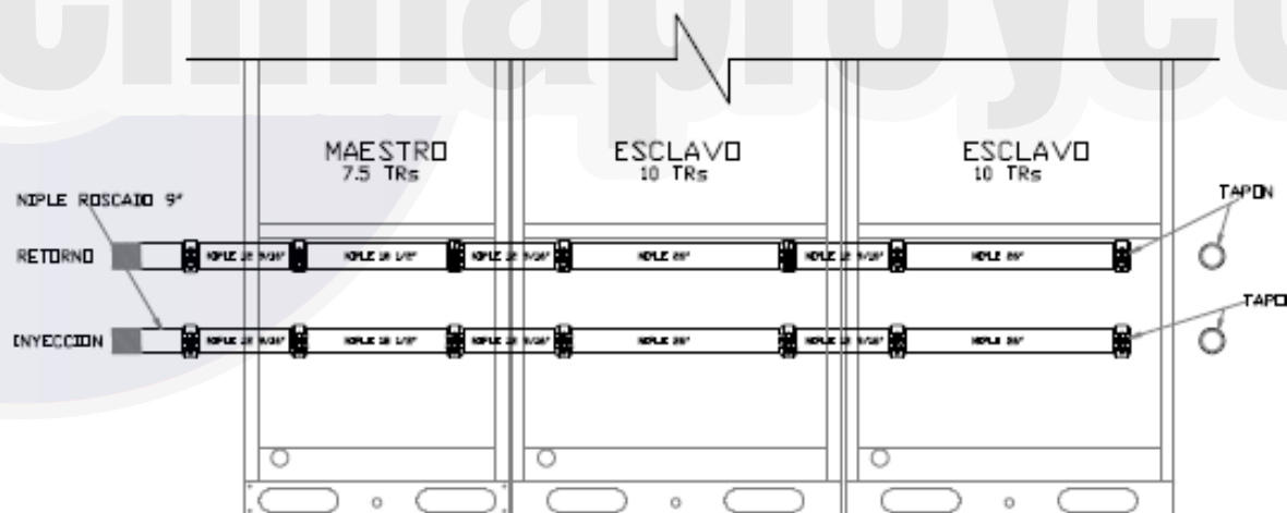
OPCION 2 DE CONEXION
