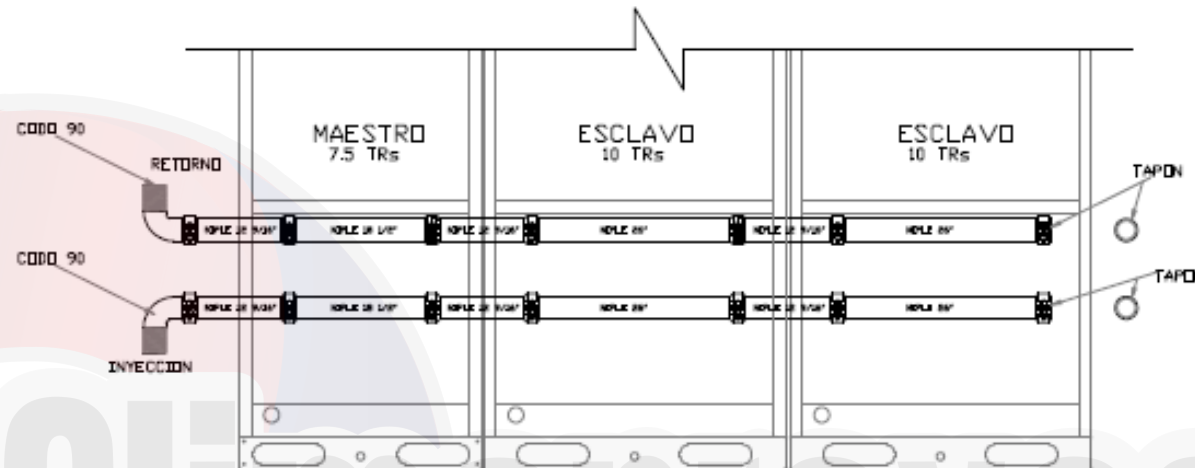
OPCION 1 DE CONEXION
