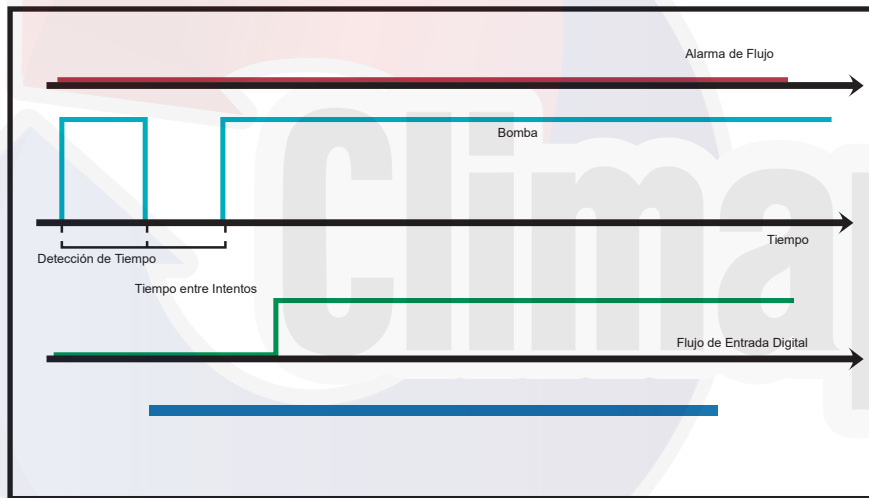
Ejemplo del ciclo de la puesta en marcha de la bomba, donde el flujo se detectó en el segundo intento
