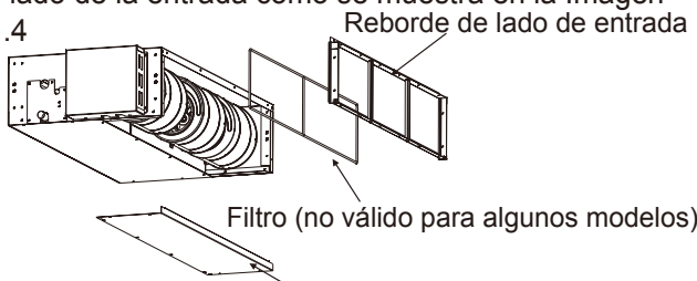
Fig. 3.1.3 Tapa de la cámara
