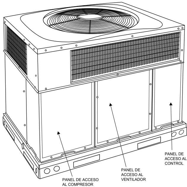
Fig. 23 – Paneles de acceso de la unidad A170032SP
