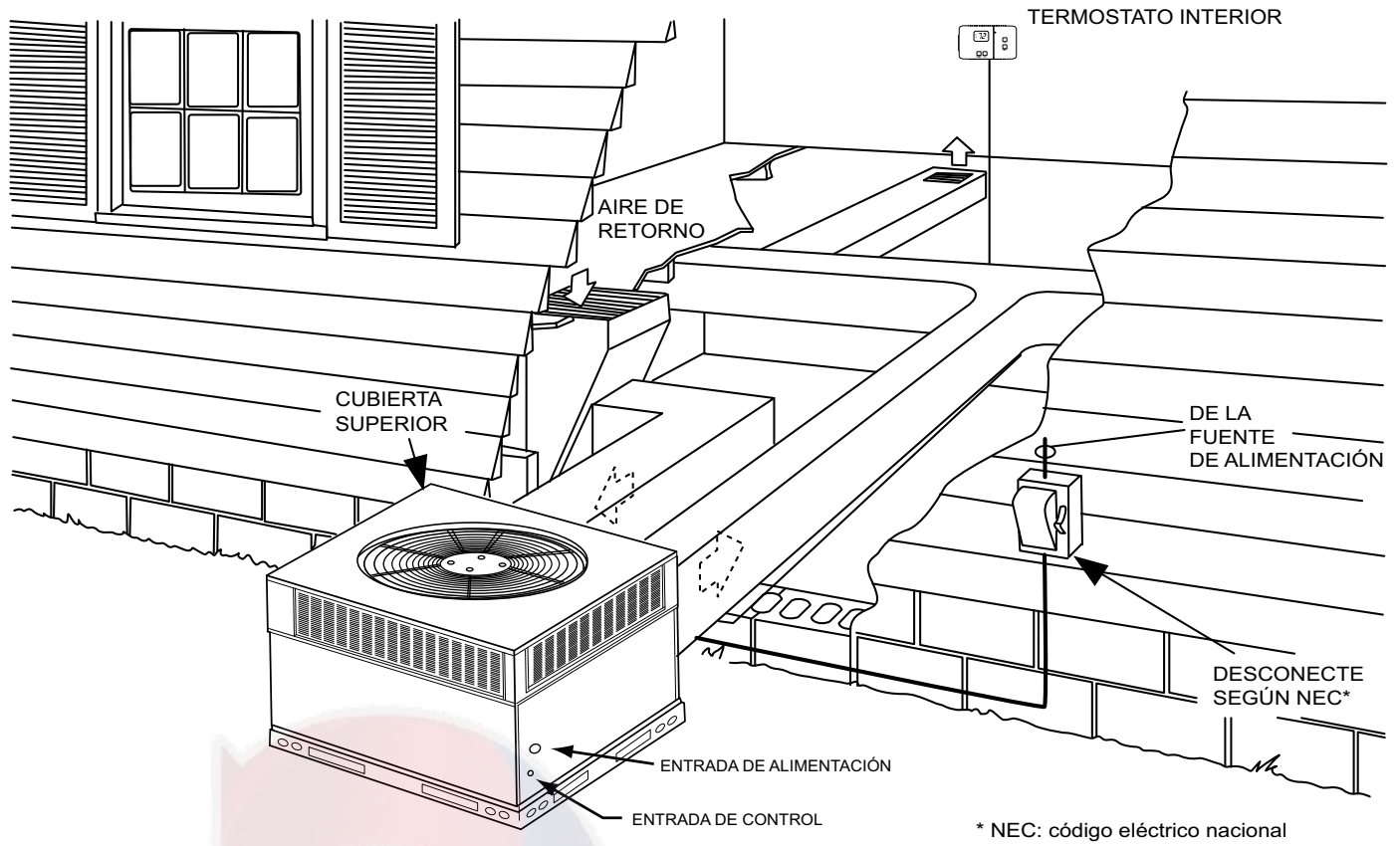
Fig. 11 – Instalación típica
