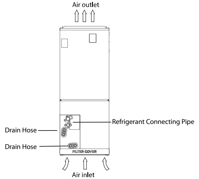
Fig. 2 — Air Handler
