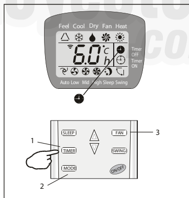
Indicador evaporadora
